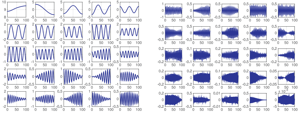
Fig. 12. T_x^i(x) .
