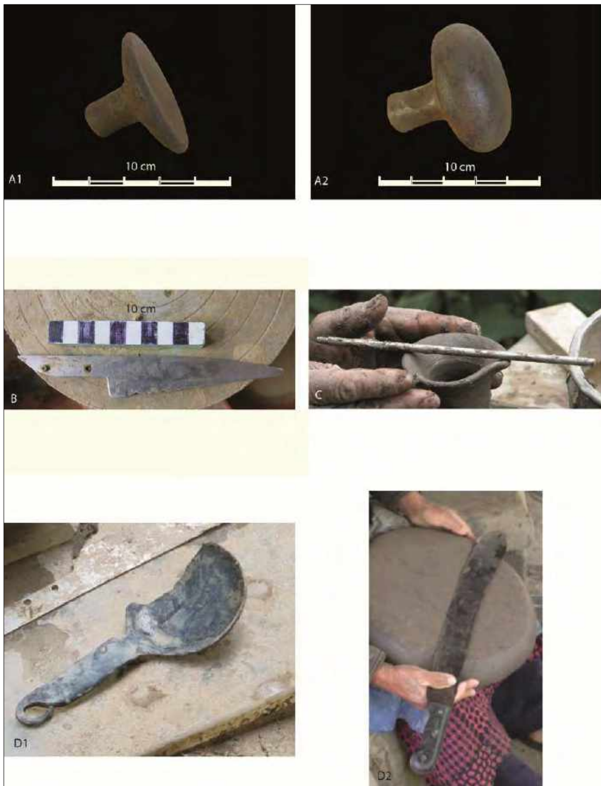
FIG. 4D 1. OUTILS DE FAÇONNAGE : Battage.- A1 : battoir ; A2 : contre-battoir. Raclage.- B : couteau. Ébauchage.- C : tige métallique (ébauchoir, Sígsig). Rabotage.- D1 : cuiller ; D2 : machette.
